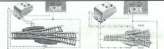
Fig. 2 Modell-Gleis PROFI-/N«piccolo»-Gleis Anschluss der Dreiwegweiche mit zwei Elektroantrieben an das Pultstellwerk.
