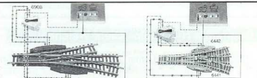
Fig. 4 Modell-Gleis PROFI-/N«piccolo»-Gleis Anschluss der Dreiwegweiche mit zwei Elektroantrieben an das Gleisbildstellwerk.
